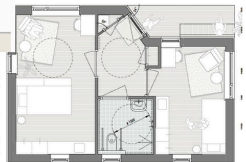
Ontwerp van het tinyhouse, bovenaanzicht
